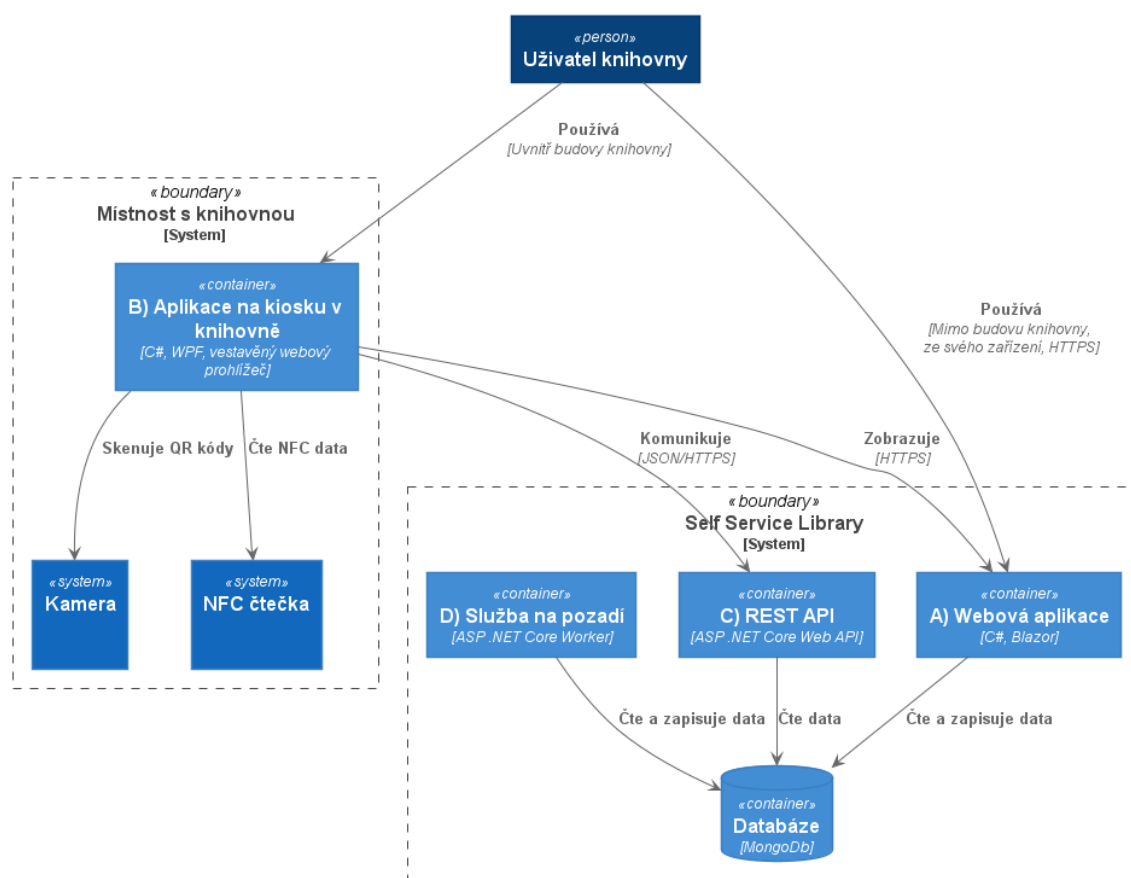
Vývojový diagram 8: Celkový kontext vytvářeného knihovního systému
