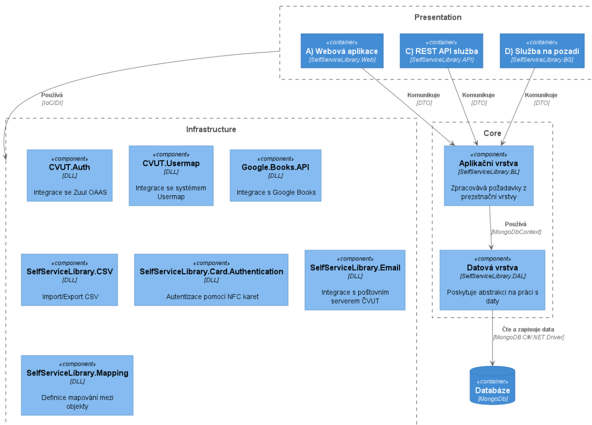
Vývojový diagram 10: Diagram rozmístění a závislostí jednotlivých komponent
